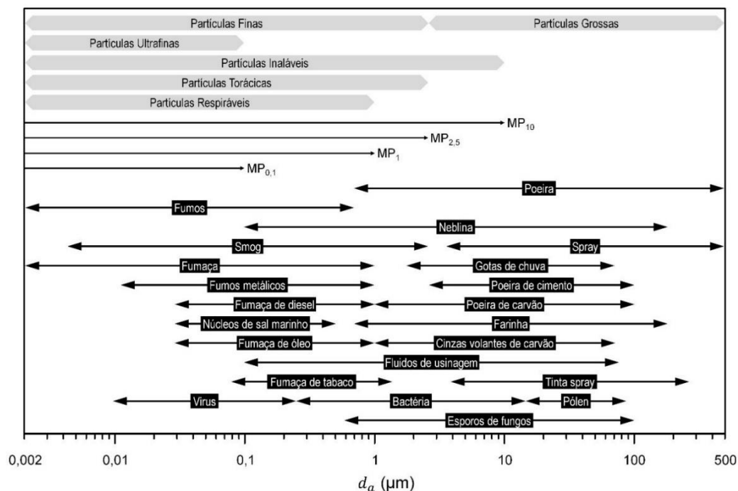
Figura 2: Os materiais particulados, suas diferentes origens e classificações.
