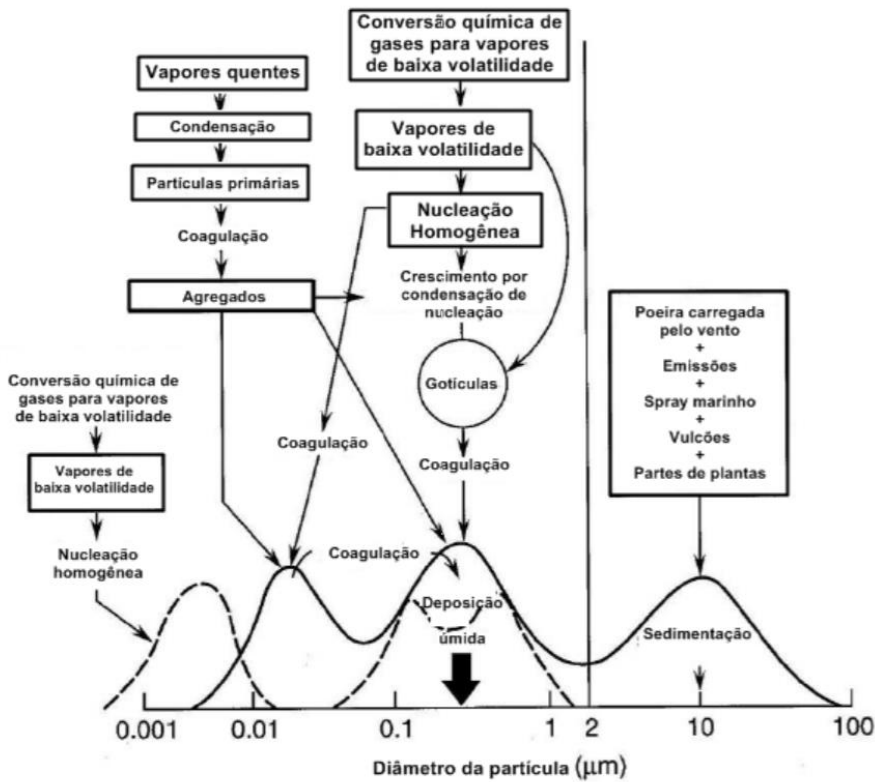
Figura 1: Distribuição Granulométrica do Aerossol Troposférico
